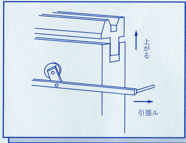
改造不可能な下ビーム
